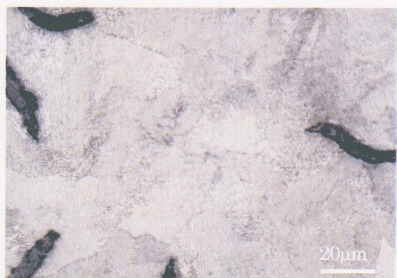
Longitudinal direction
